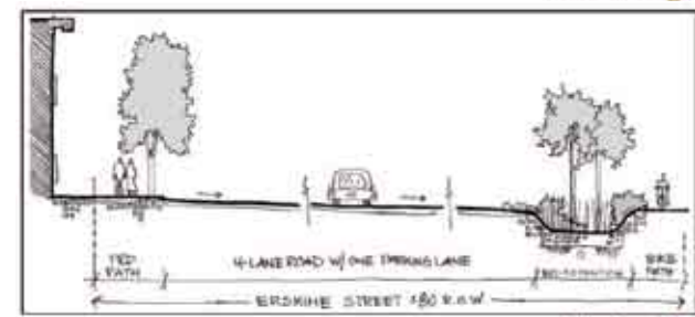
Erskine Street Section = N.T.S.
