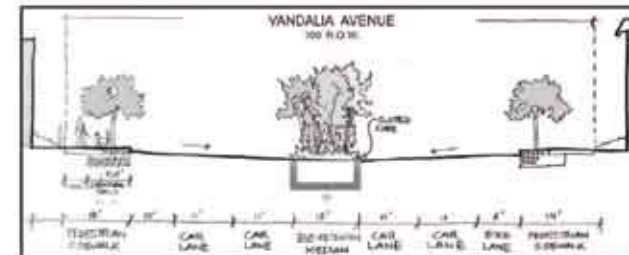
Vandalia Avenue Section = N.T.S.
