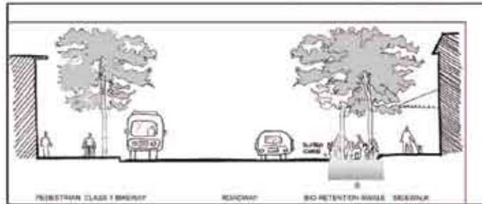
Elton Street Section = N.T.S.
