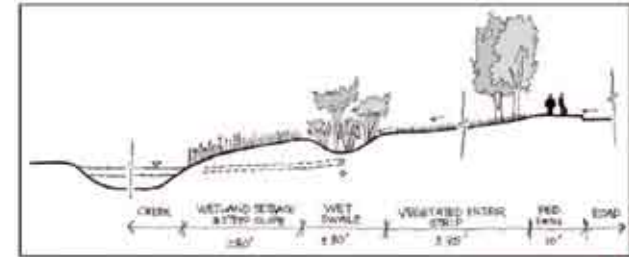
Hendrix Creek Park Section = N.T.S.
